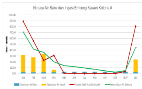
Gambar 6. Neraca air embung kawari kriteria A
